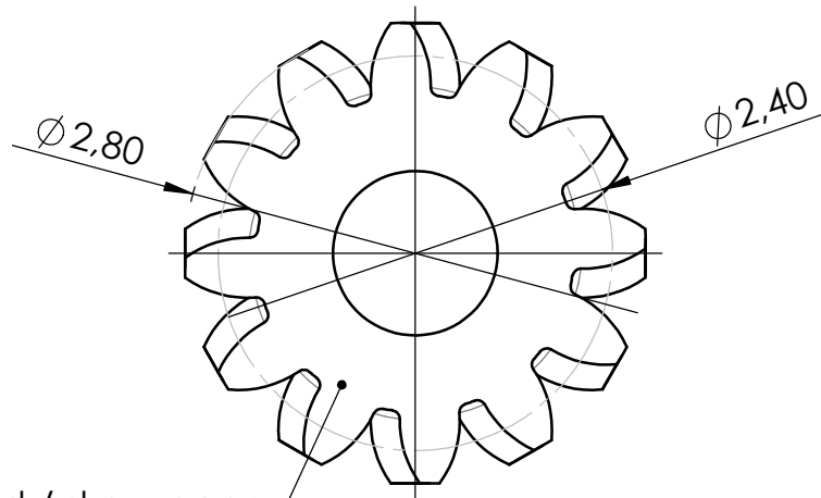
Schneckenrad / skew gear z=12 / m=0,2
