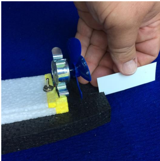
Das Ruderblatt im Spalt am Heck einstecken
