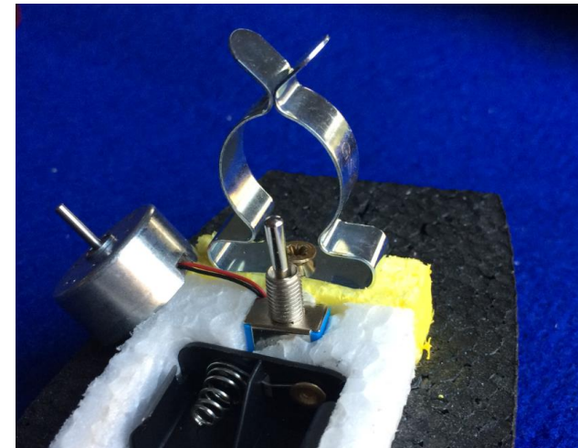
Die Klammer erwartet den Motor
