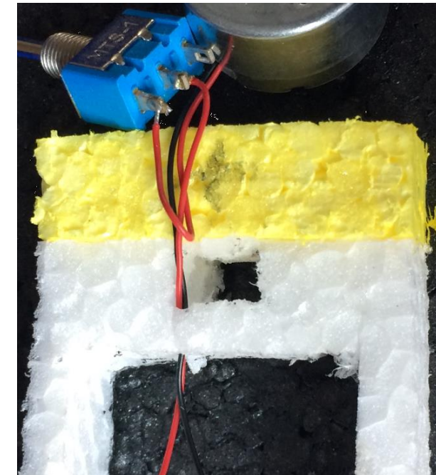
Einlegen vom Kabel in den Spalt einlegen
